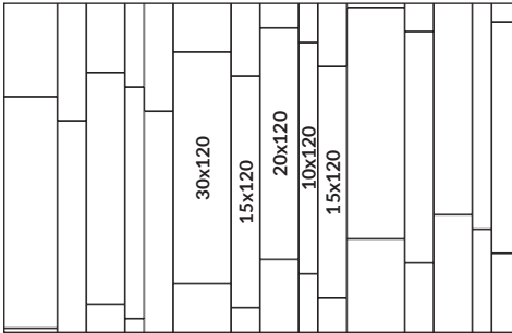
Multi 1 laying example Ejemplo de colocación Multi 1
